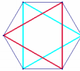
Estrella 6/2 (hexagrama)
